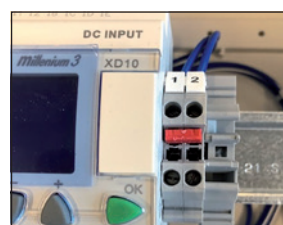
(Pont de fil pour configuration gravitaire)
