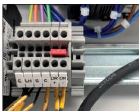
(Pont de fil pour contourner la sécurité de la porte)
